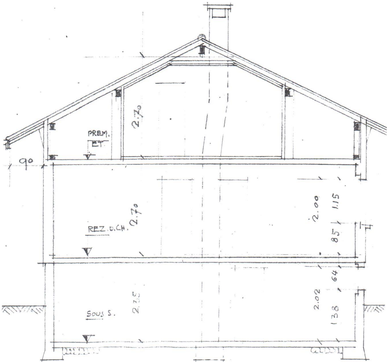
COUPE.
